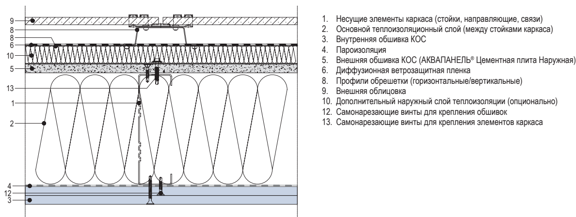
Рис. 2. Основные компоненты наружной каркасно-обшивной стены
