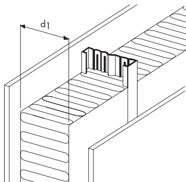
Рис. 14. Толщина утепляющего слоя наружной КОС с применением ЛСТК
