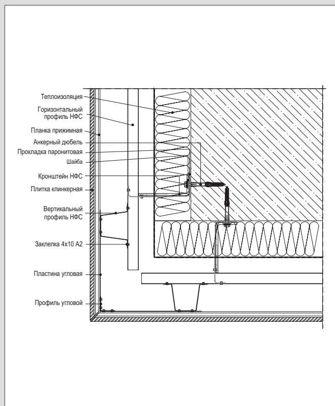
А 3 – WM 111 (4а 100) С. Горизонтальный разрез внешнего угла по перекрытию
