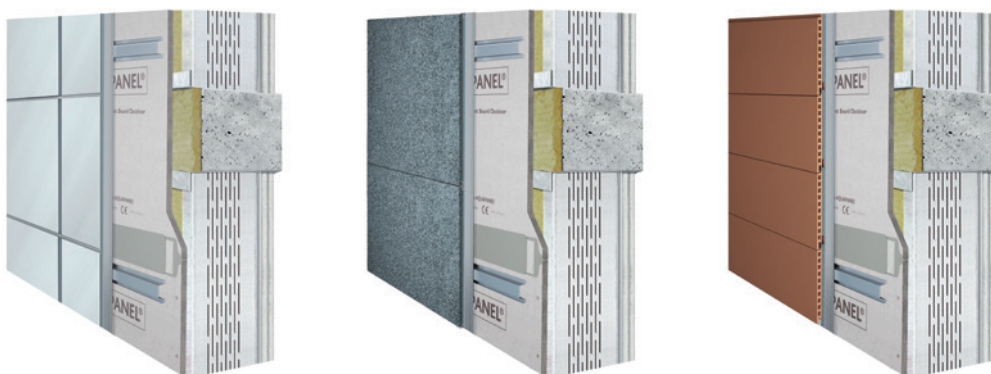
Рис. 4. Виды фасадных облицовок КОС
