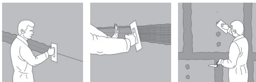
Рис. 24. Шпаклевание стыков и мест установки шурупов
