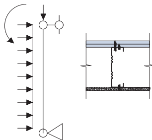
Рис. 11. Расчетная схема стойки каркаса стены при воздействии ветровой нагрузки и от собственного веса фасада, схема раскрепления полок стойки термопрофиля обшивками КОС
