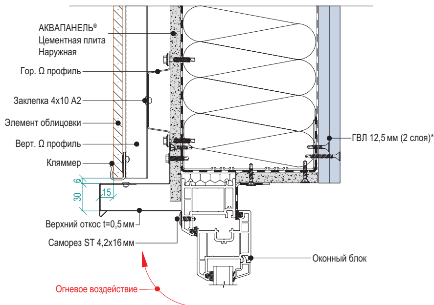
Рис. 8а. Пример узла верхнего откоса с противопожарной отсечкой пламени огня
