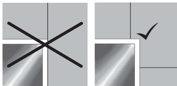
Рис. 23. Крепление плит в области проема
