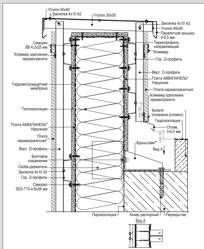
D 4 – WM 112 (2) С. Крепление к плите покрытия. Паранет
