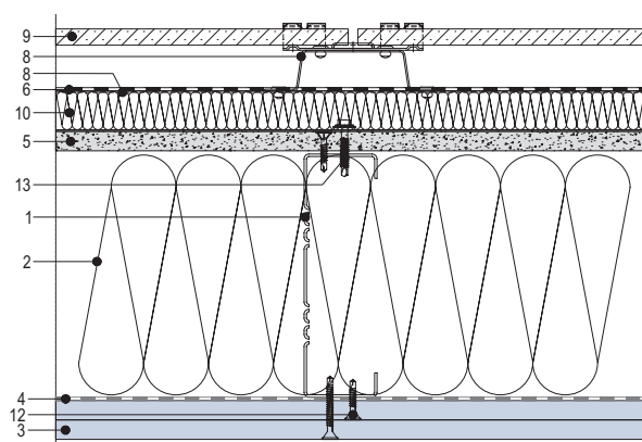
Рис. 8. Тип № 3. Схема конструктивного исполнения наружной несущей КОС с зазором и дополнительным наружным утеплением (расшифровку цифровых обозначений см. в табл. 1)
