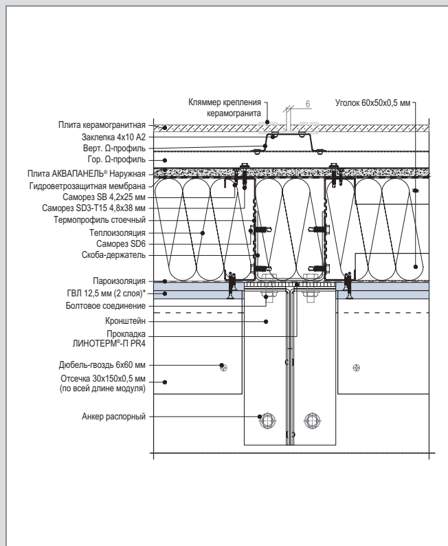
D 2 – WM 112 (2) С. Горизонтальный разрез рядового модуля. Крепление к перекрытию
