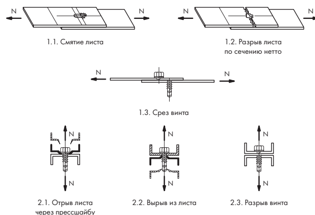
Рис. 12. Графическое изображение типов отказа соединений тонкостенных конструкций на саморезах
