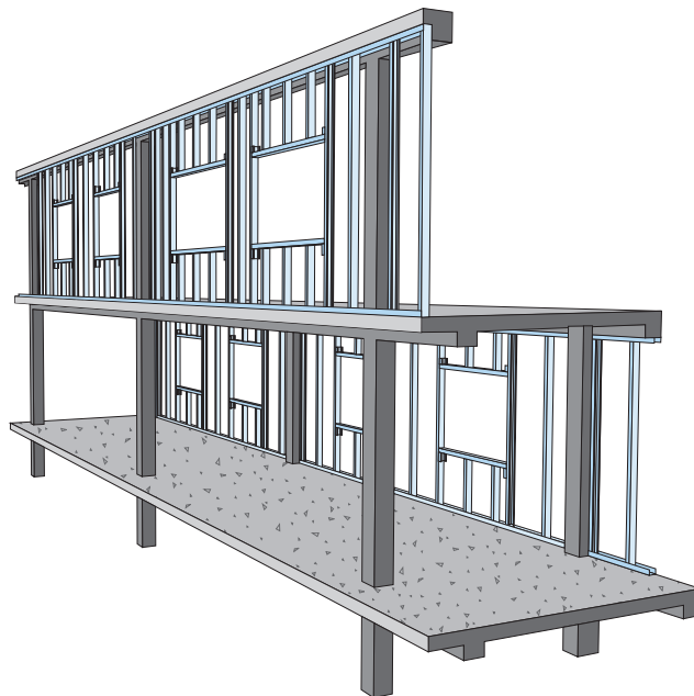
Рис. 3. Схематическое изображение несущих КОС с каркасом из ЛСТК (класс А или В) в здании с несущим монолитным железобетонным каркасом
