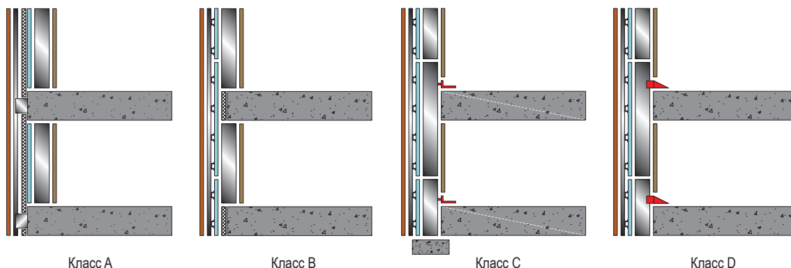
Рис. 5. Классификация наружных ненесущих стен в зависимости от типа примыкания к несущим конструкциям здания
