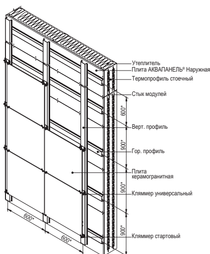
Рис. 1. Общий вид наружной каркасно-обшивной стены (КОС) с каркасом из ЛСТК
