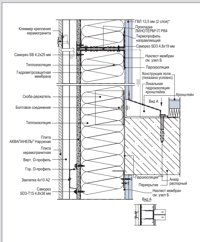
D 1 – WM 112 (2) С. Вертикальный разрез рядового модуля. Крепление к перекрытию
