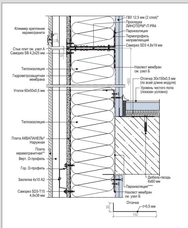
D 3 – WM 112 (2) С. Вертикальный разрез рядового модуля
