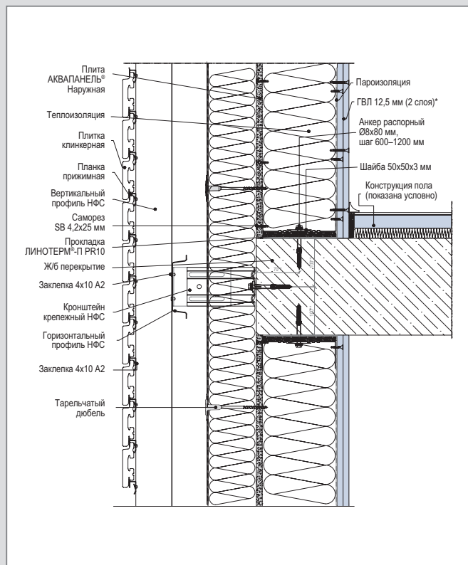
А 1 – WM 111 (4а 100) С. Вертикальный разрез рядового модуля. Примыкание к перекрытию
