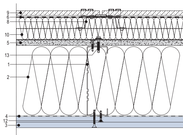
Рис. 9. Тип № 4. Схема конструктивного исполнения наружной несущей КОС с зазором и дополнительным наружным утеплением (расшифровку цифровых обозначений см. на рис. 2)
