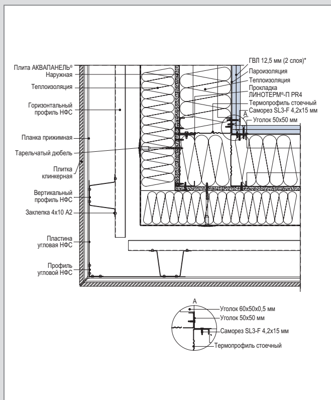
А 2 – WM 111 (4а 100) С. Горизонтальный разрез внешнего угла
